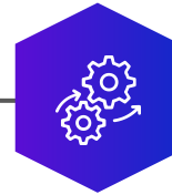
QA Automation
